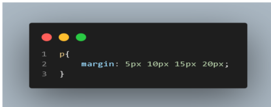
Gambar 3.74 Margin dengan shorthand
