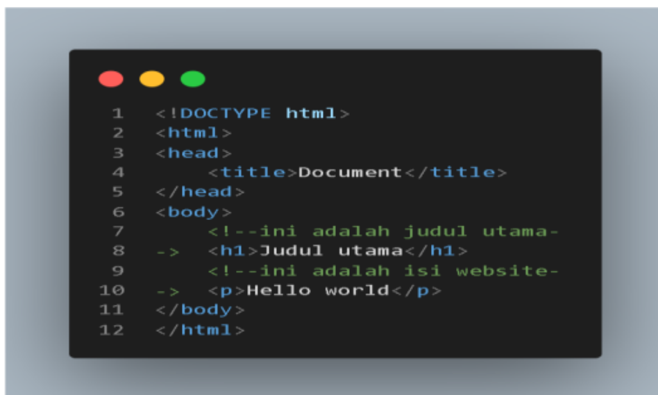
Gambar 2.5 Komentar html
