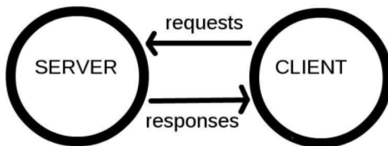
Gambar 1.3 pemanggilan website
