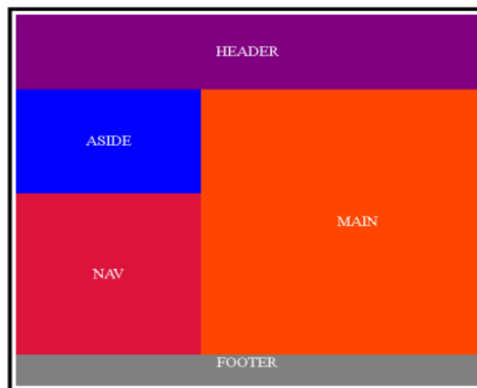
Gambar 2.37 Struktur Website
