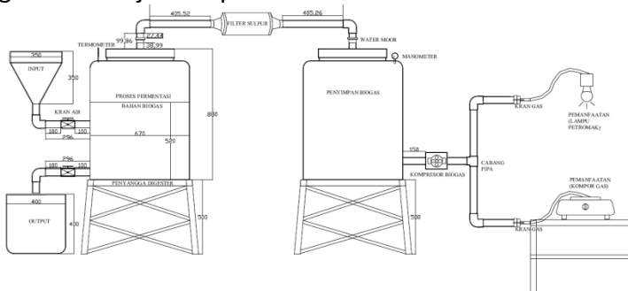
Gambar 3. Rancangan Biodigester
