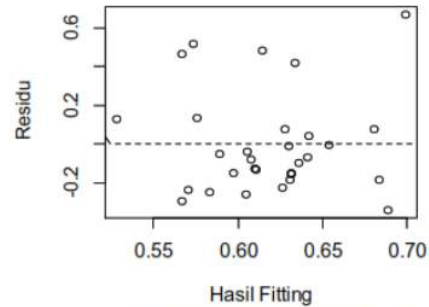
Gambar 3. Plot Residu VS Hasil Estimasi
