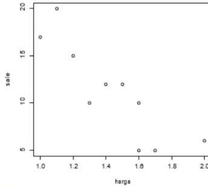
Gambar 1. Plot Penjualan
