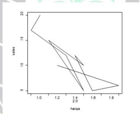
Gambar 2. Plot Penjualan dengan Fungsi Tambahan Lines
