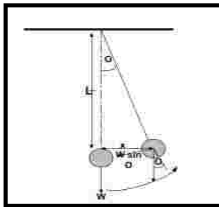
Gambar 4.7. Sistem Bandul
