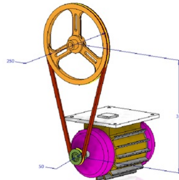
Gambar 2. Desain Sistem Penggerak Trainer
