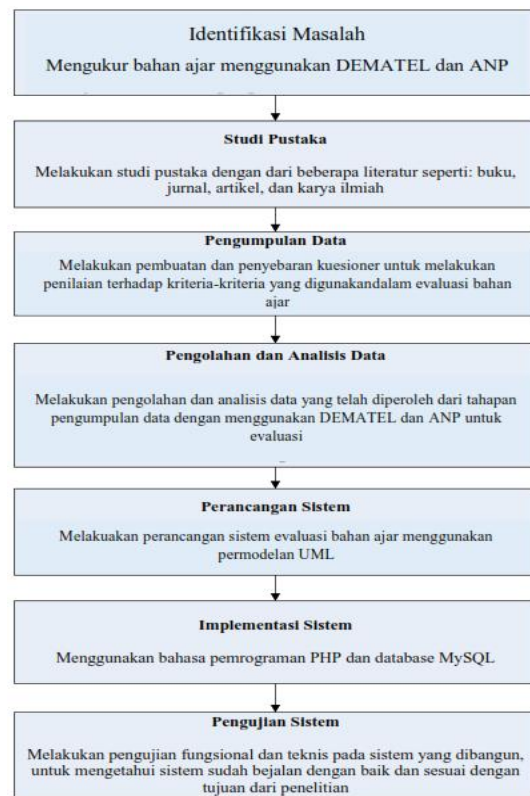
Gambar 2. Metodologi Penelitian
