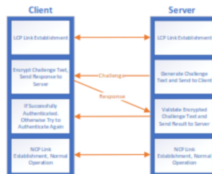
Gambar 3. Skema MS-CHAP
