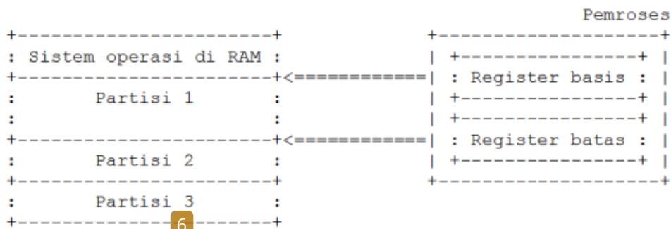
Gambar 6.6 Skema relokasi dan proteksi menggunakan register basis dan register batas
