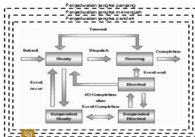
Gambar 3.1 Tipe-tipe penjadwalan dikaitkan dengan diagram state
