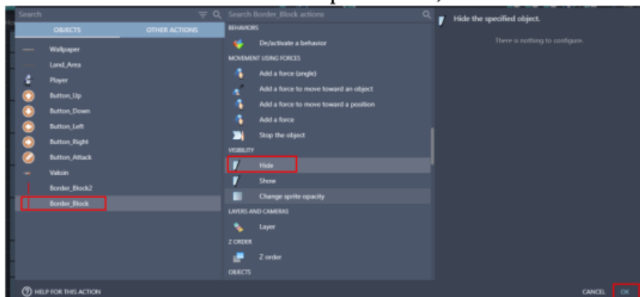
Gambar 1. 47 Memilih Hide pada Objek Border_Block
