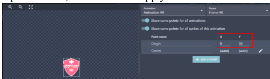
Gambar 6. 55 Mengatur Value X dan Y pada Shield_HS
