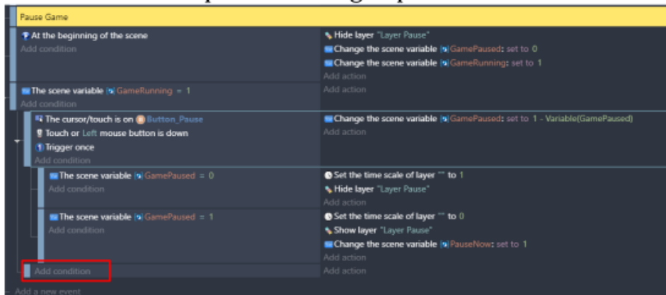
Gambar 4. 53 Memilih Add Condition
