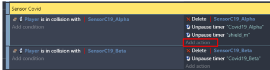
Gambar 6. 63 Memilih Add Action
