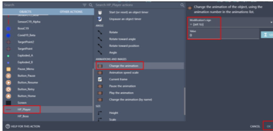
Gambar 5. 29 Memilih Change the Animation
