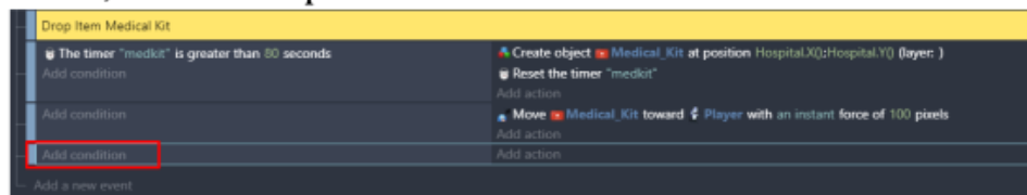
Gambar 6. 94 Memilih Add Condition
