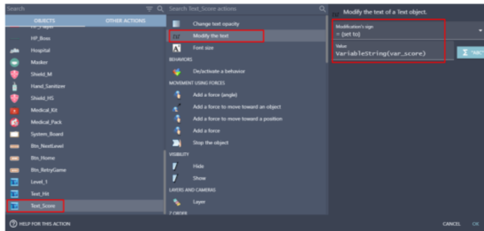
Gambar 7. 30 Memilih Modify the Text pada Text_Score
