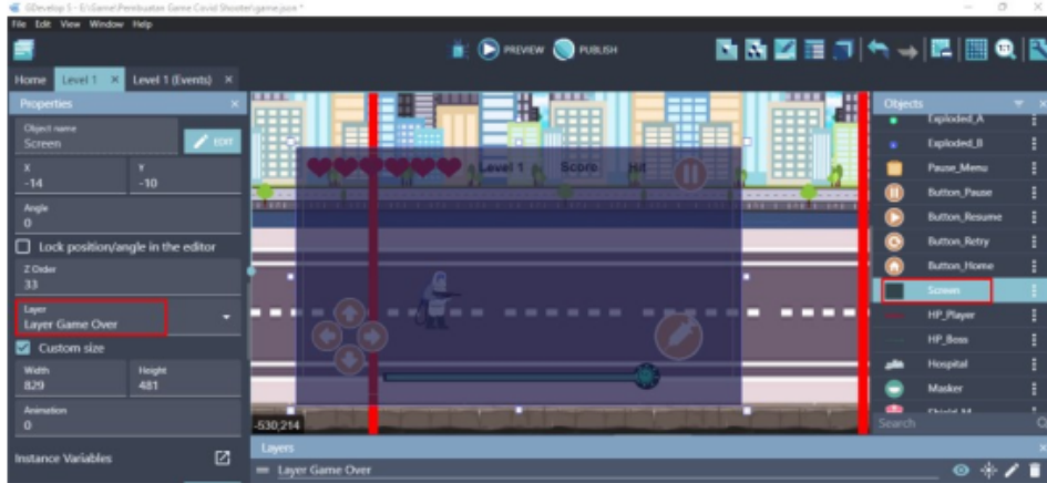
Gambar 7. 38 Menambahkan Screen ke Layer Game Over
