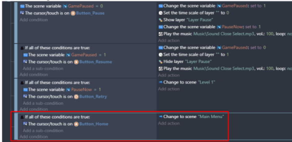
Gambar 4. 97 Hasil Pembuatan Sistem Home
