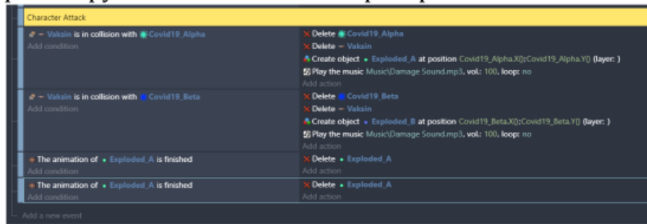
Gambar 3. 29 Melakukan Duplikasi Program Exploded_A
