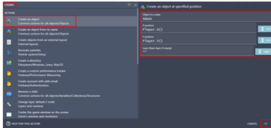
Gambar 1. 16 Menambahkan Fungsi Create an Object
