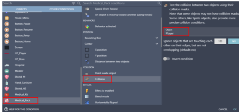
Gambar 6. 76 Memilih Collision pada Medical_Pack
