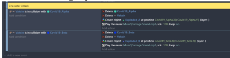
Gambar 3. 24 Mengubah Hasil Duplikasi Program Pada Covid19_Alpha Menjadi Covid19_Beta
