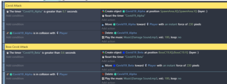
Gambar 3. 40 Duplikasi Program Serangan Covid19_Alpha
