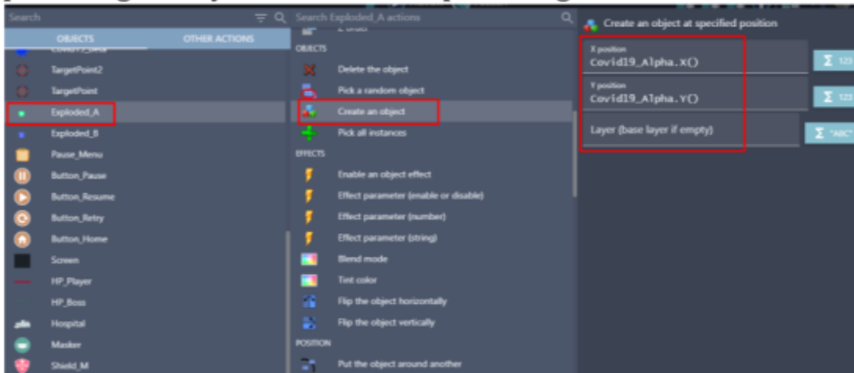
Gambar 6. 37 Memilih Create an Object
