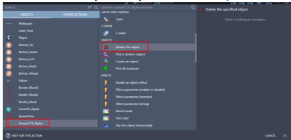
Gambar 2. 31 Memilih Delete the Object pada SensorC19_Alpha
