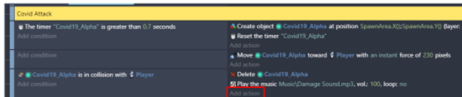
Gambar 5. 56 Memilih Add Action
