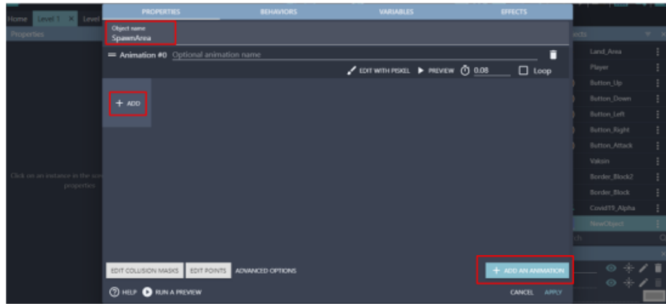
Gambar 2. 7 Menambahkan Objek Spawn Area
