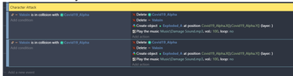
Gambar 3. 23 Melakukan Duplikasi Program Covid19_Alpha
