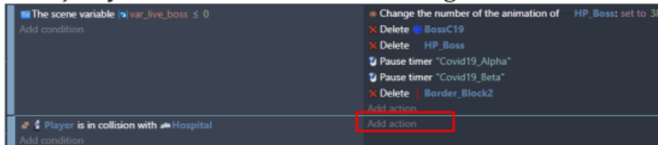
Gambar 7. 95 Memilih Add Action
