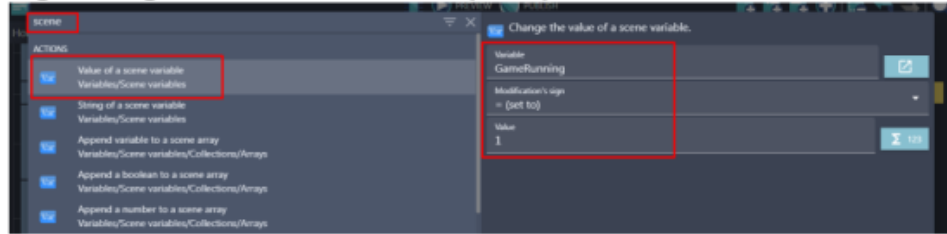
Gambar 4. 37 Memilih Value of a Scene Variable
