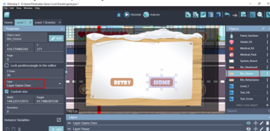
Gambar 7. 41 Menambahkan Btn_Home pada Scene Level 1
