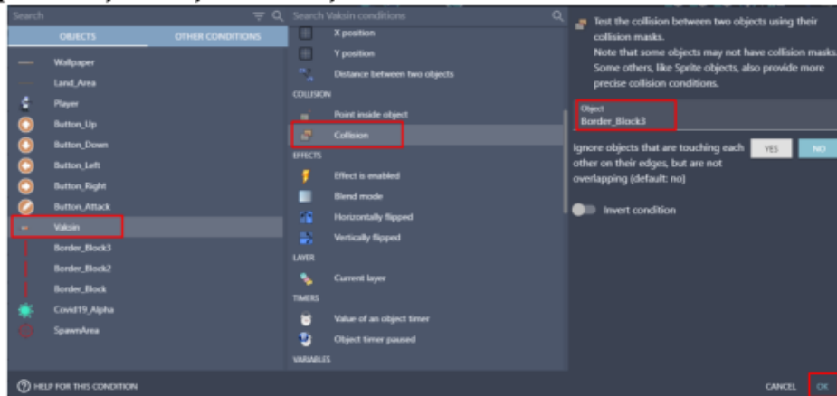
Gambar 1. 51 Memilih Collision pada Vaksin Terhadap Objek Border_Block3
