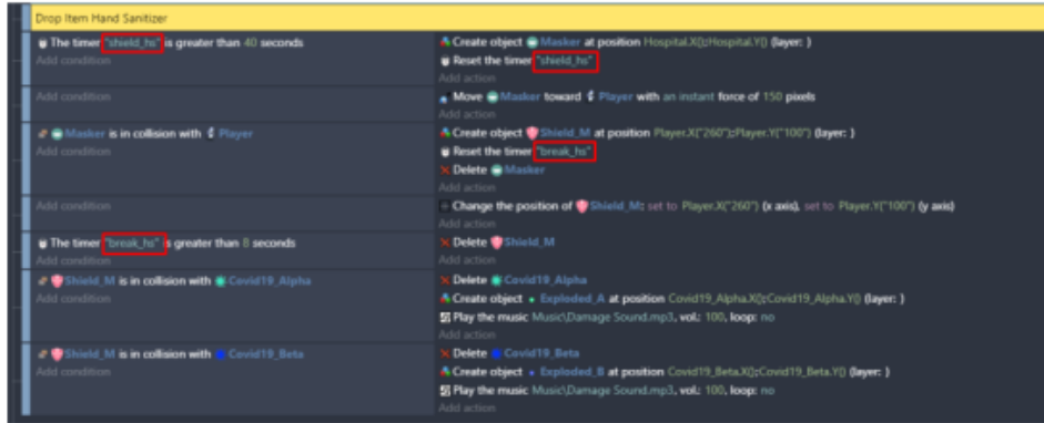
Gambar 6. 58 Modifikasi Variabel pada Drop Item Hand Sanitizer
