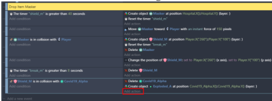
Gambar 6. 38 Memilih Add Action
