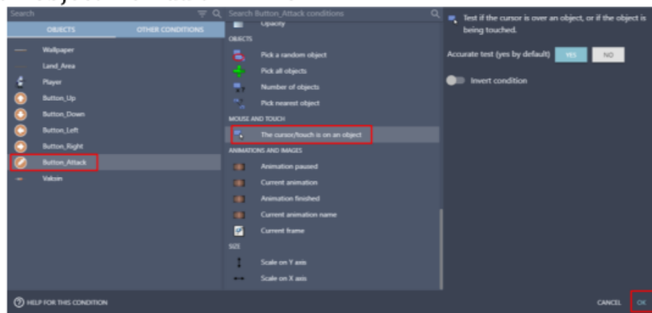
Gambar 1. 11 Menambahkan Fungsi Touch Pada Button_Attack
