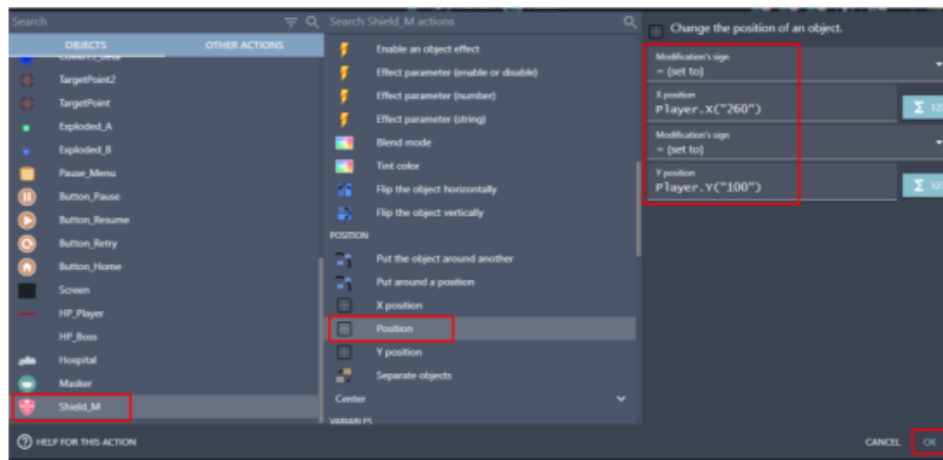
Gambar 6. 29 Menambahkan Position Shiled_M pada Player
