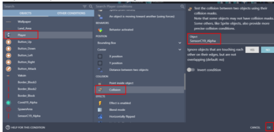
Gambar 2. 30 Menambahkan Collision Pada Player
