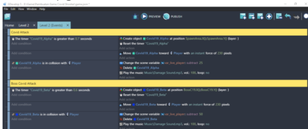
Gambar 8. 11 Pengembangan Pada Serangan Karakter Musuh
