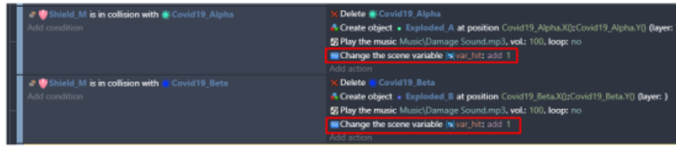
Gambar 7. 36 Duplikasi var_hit pada Drop Item Masker
