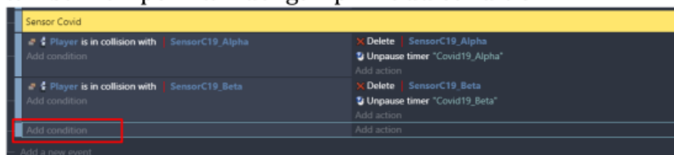
Gambar 2. 66 Memilih Add Condition
