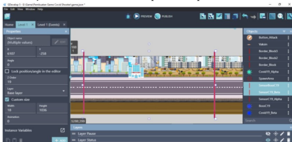
Gambar 2. 50 Menambahkan Sensor ke Dalam Scene Level 1
