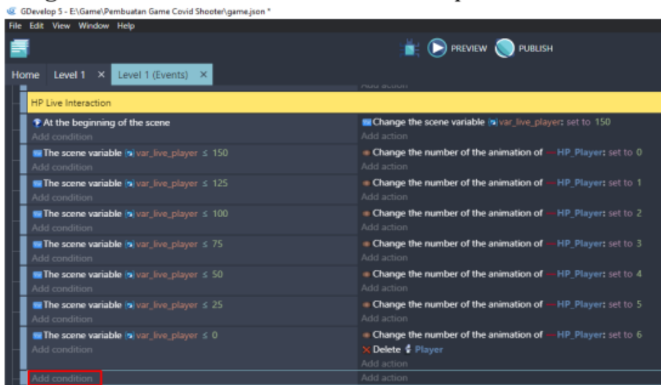
Gambar 5. 26 Memilih Add Condition
