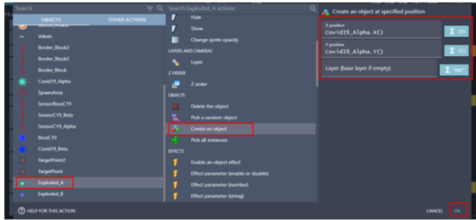
Gambar 3. 19 Memilih Create an Object Pada Objek Exploded_A
