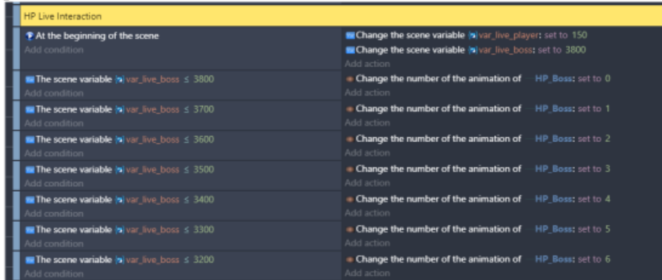
Gambar 5. 39 Modifikasi Program HP_Boss
