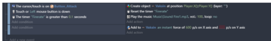
Gambar 1. 23 Hasil Pembuatan Program Button_Attack
