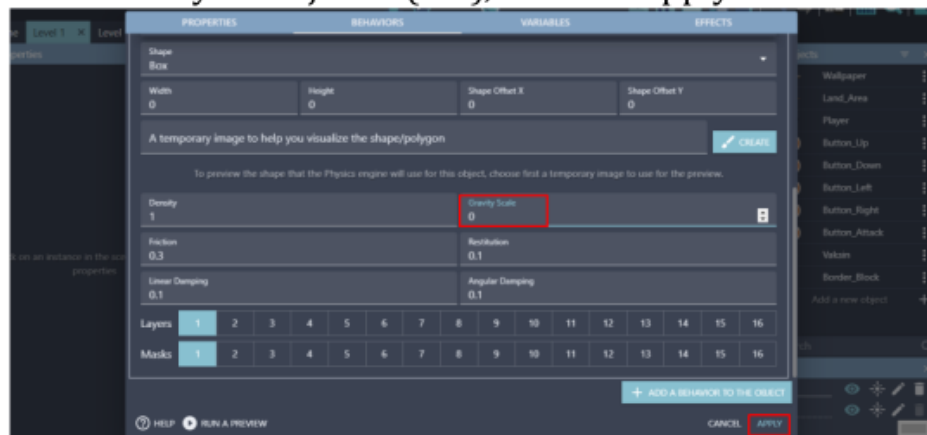
Gambar 1. 38 Mengatur Gravity Scale pada Physics engine 2.0
