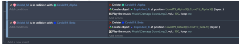
Gambar 6. 41 Modifikasi Program Collision Shield_M
