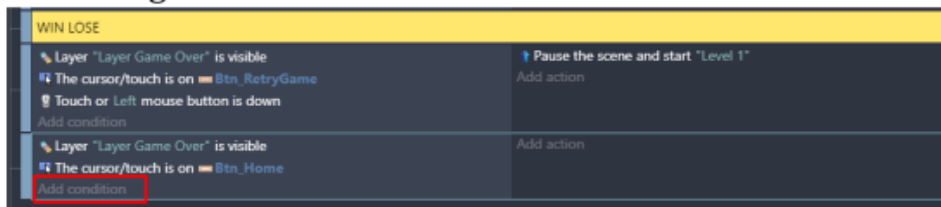
Gambar 7. 57 Memilih Add Condition
