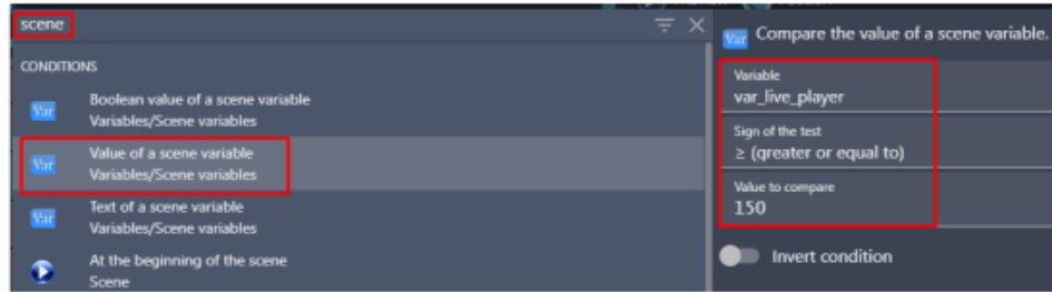
Gambar 5. 27 Memilih Value of a Scene Variable
