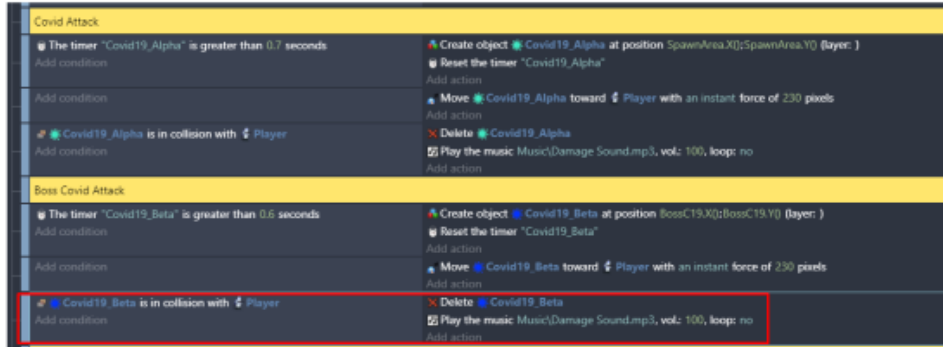
Gambar 3. 41 Mengubah Covid19_Alpha Menjadi Covid19_Beta
