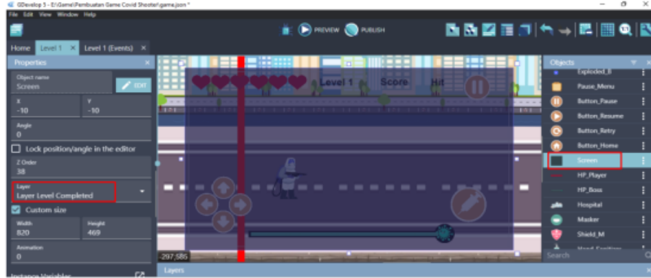
Gambar 7. 65 Menambahkan Screen ke Scene Level 1
