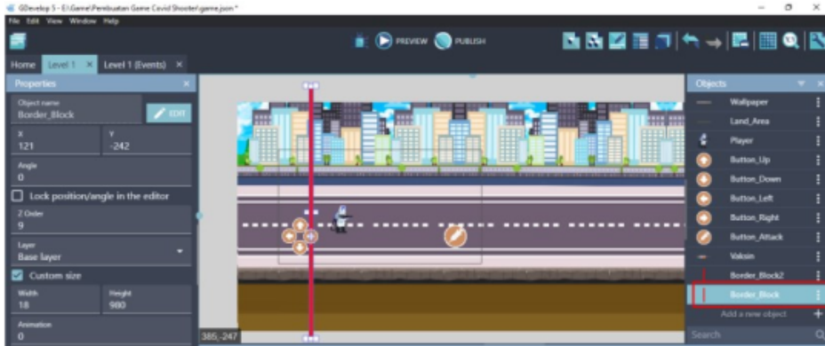
Gambar 1. 40 Mengatur Border_Block ke Dalam Scene Level 1
