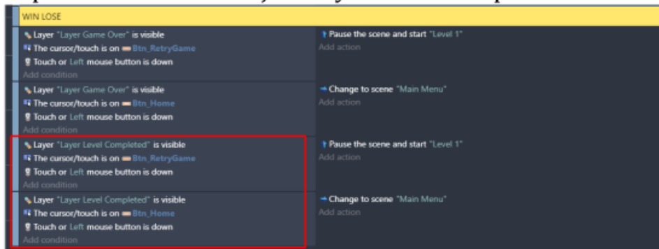
Gambar 7. 87 Modifikasi Menjadi Layer Level Completed
