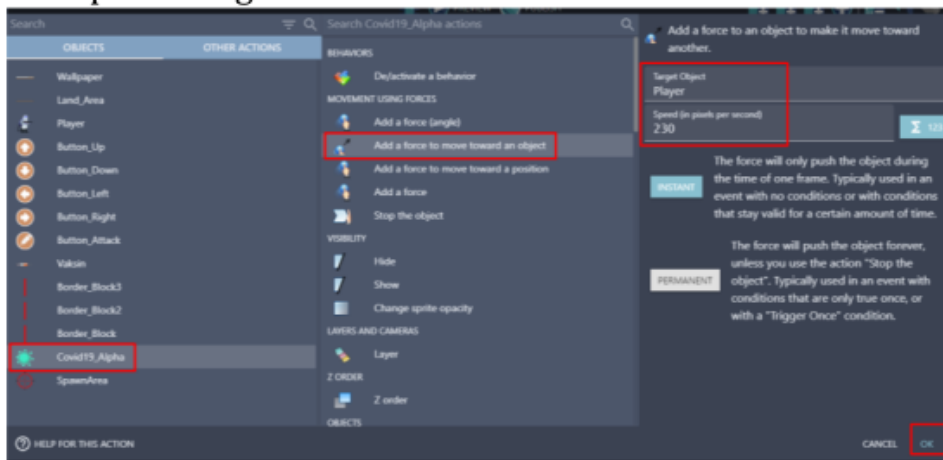
Gambar 2. 22 Memilih Add a Force to Move Toward an Object pada Covid19_Alpha
