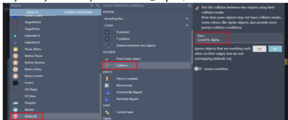
Gambar 6. 34 Memilih Collision pada Shield_M
