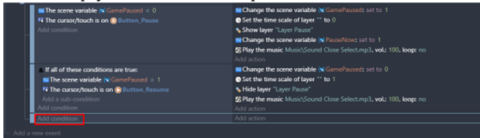
Gambar 4. 83 Memilih Add Condition
