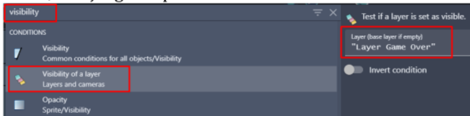
Gambar 7. 54 Memilih Visibility of a Layer
