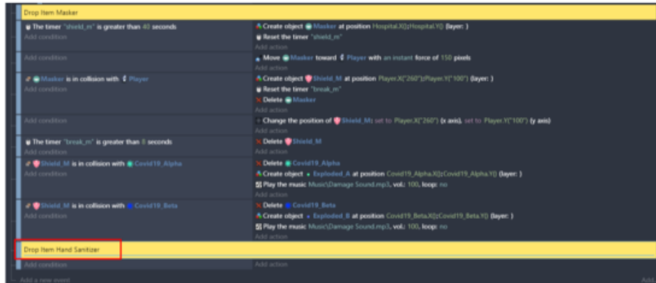
Gambar 6. 56 Menambahkan Comment Drop Item Hand Sanitizer
