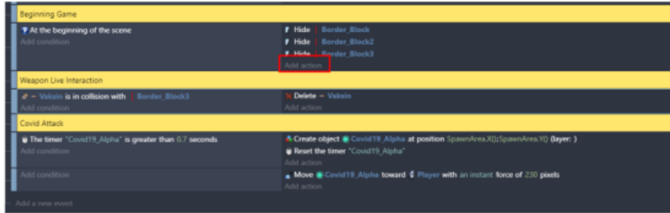
Gambar 2. 23 Memilih Add Action
