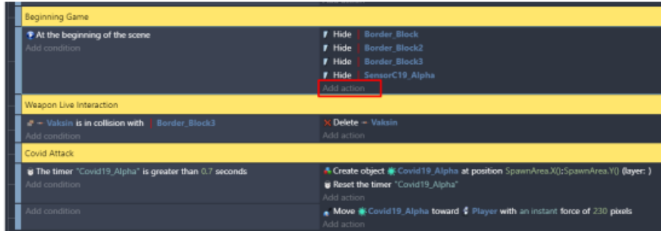
Gambar 2. 25 Memilih Add Action
