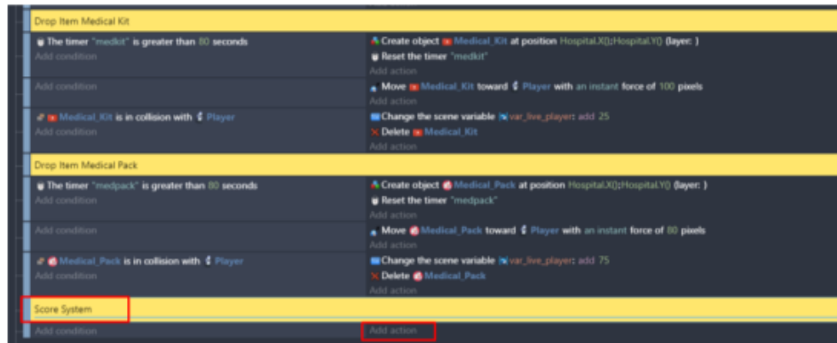
Gambar 7. 27 Menambahkan Comment Score System
