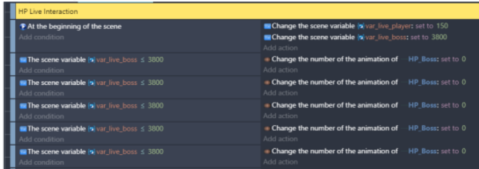
Gambar 5. 38 Duplikasi Program HP_Boss
