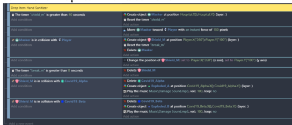
Gambar 6. 57 Duplikasi Program Masker untuk Hand Sanitizer
