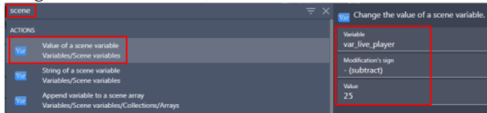
Gambar 5. 57 Memilih Value of a Scene Variable
