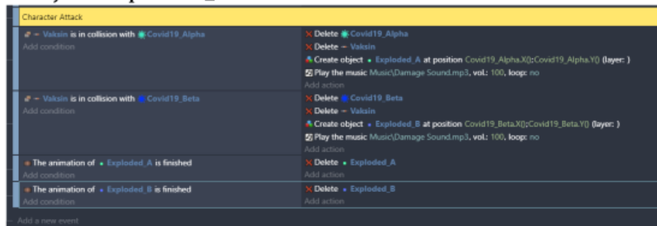
Gambar 3. 30 Mengubah Exploded_A Menjadi Exploded_B
