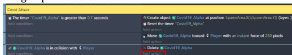
Gambar 3. 37 Memilih Add Action
