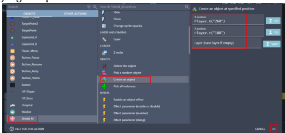
Gambar 6. 24 Memilih Create an Object
