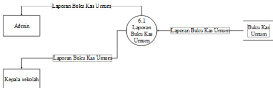
Gambar 5. DFD Level 2 Laporan Buku Kas Umum
