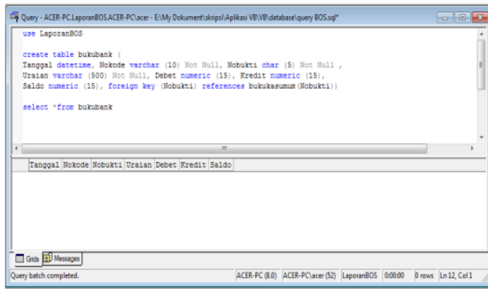
Gambar 12. Pembuatan tabel bukubank
