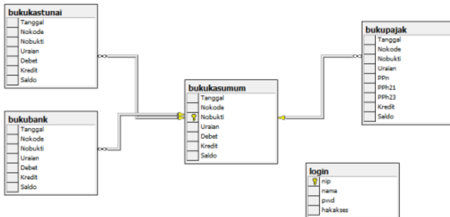
Gambar 15. Relasi Antar Tabel
