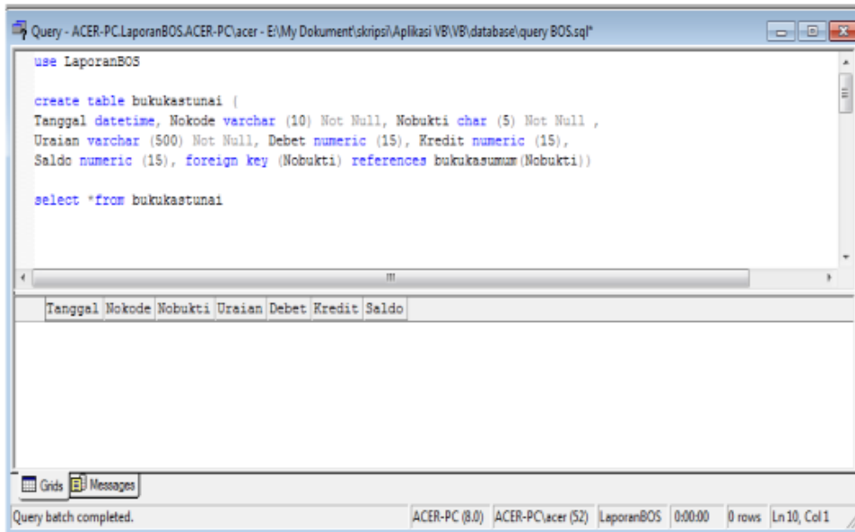
Gambar 11. Pembuatan tabel bukukastunai
