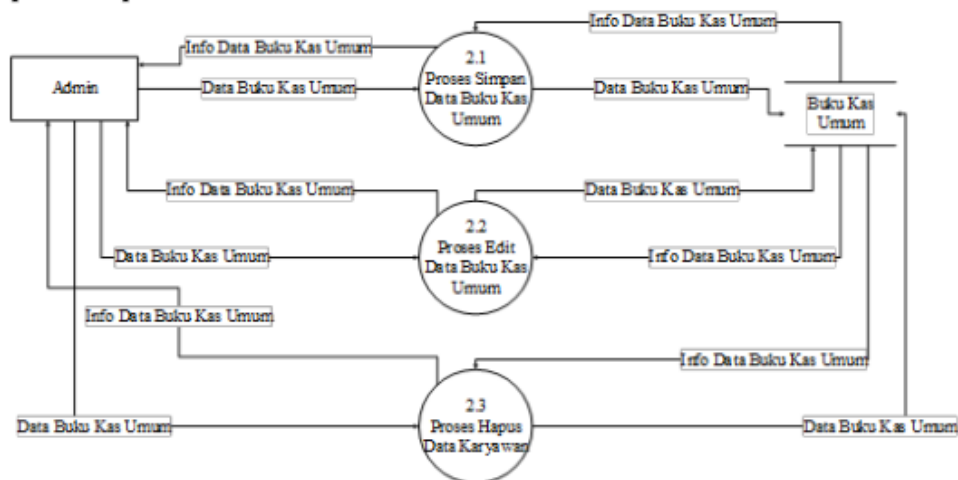
Gambar 4. DFD Level 2 Data Buku Kas Umum
