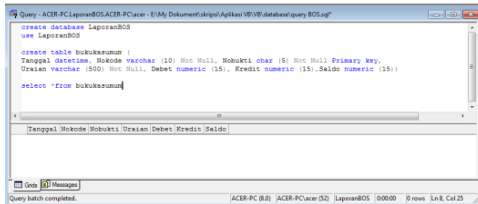
Gambar 10. Pembuatan database LaporanBOS & tabel bukukasumum
