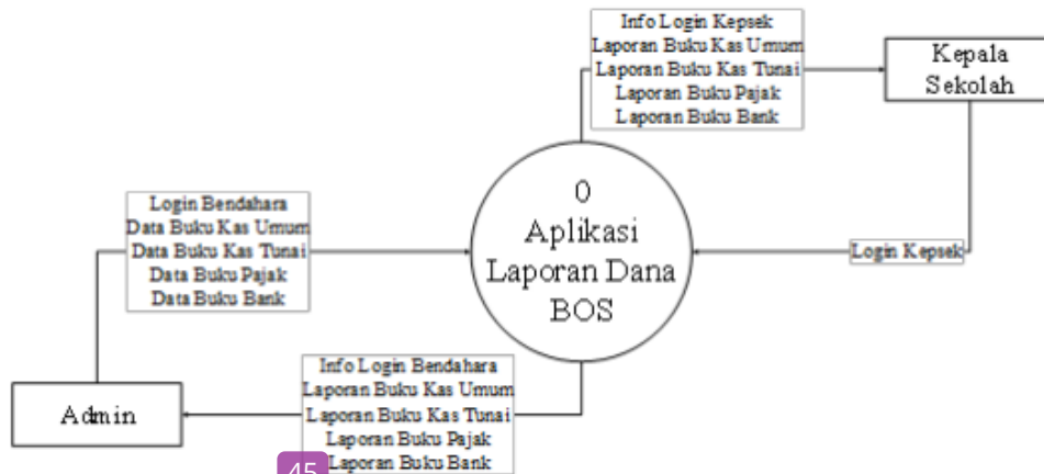
45 Gambar 2. Diagram Konteks
