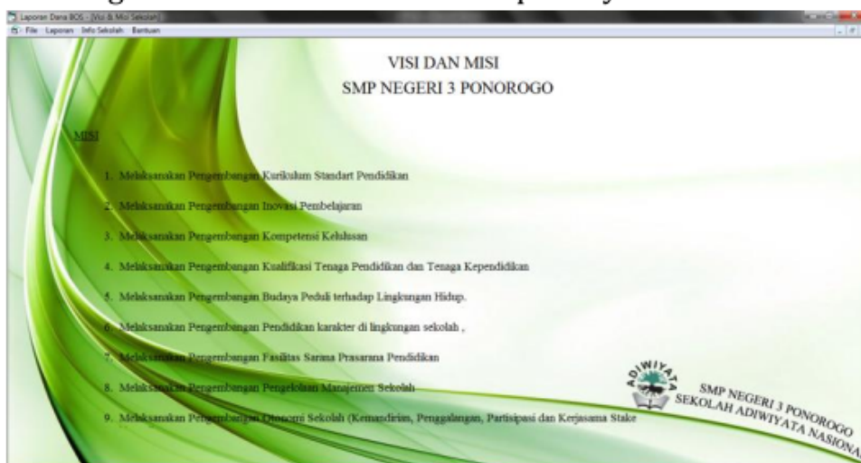
Gambar 37. Halaman misi
