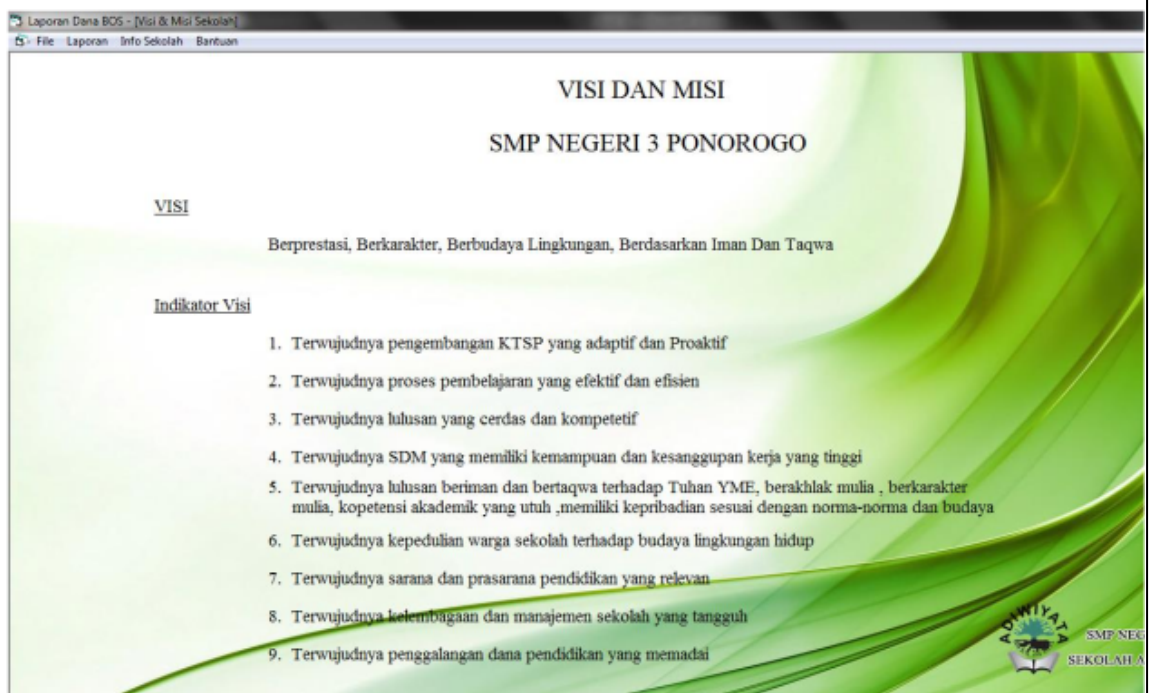
Gambar 36. Halaman visi
