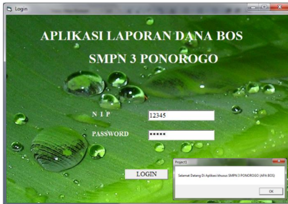
Gambar 16. Halaman Login
