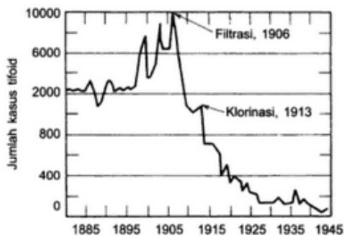
Gambar Kejadian munculnya demam tifoid di Philadelphia, 1880-1945, memperlihatkan pengaruh filtrasi dan klorinasi.
