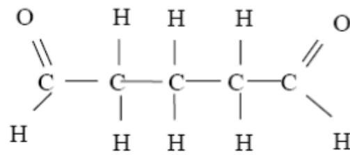
Gambar 2 Mekanisme glutaraldehid
