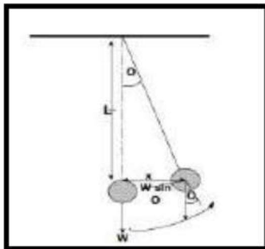
Gambar 4.7. Sistem Bandul
