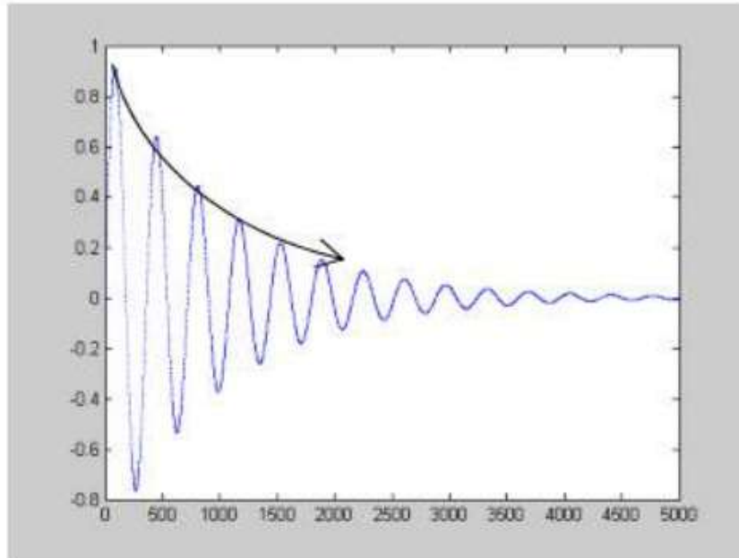
Gambar 4.5. Anatomi Gerak Harmonik Teredam
