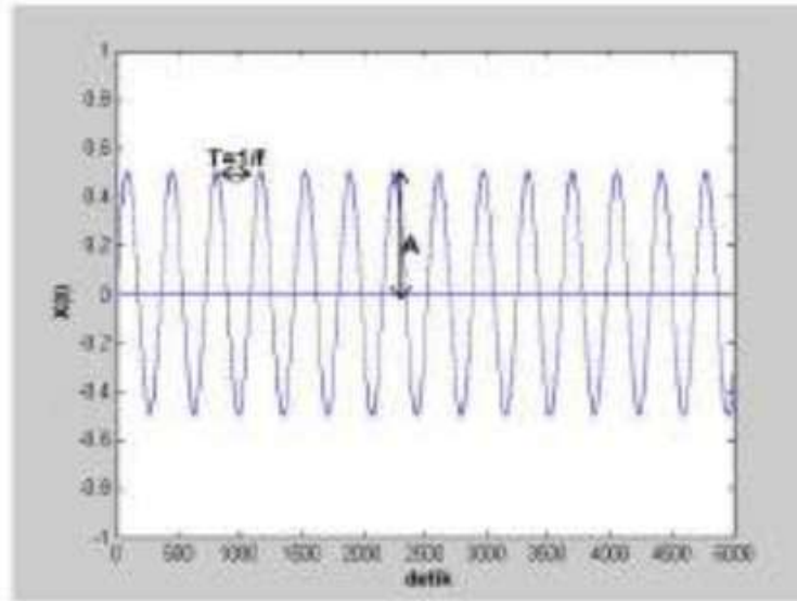
Gambar 4.6. Anatomi Periode, Frekuensi dan Amplitudo
