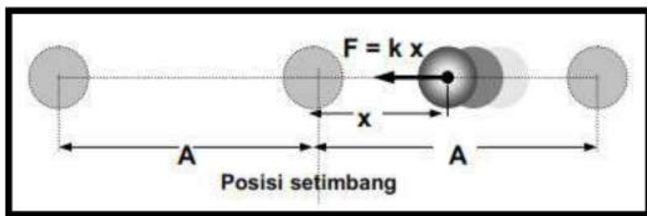
Gambar 4.3. Anatomi Gerak Harmonik Sederhana
