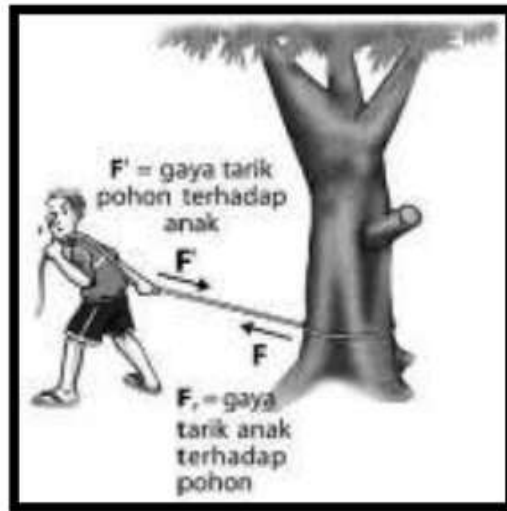
Gambar 4.10. Penerapan Hukum Newton III
