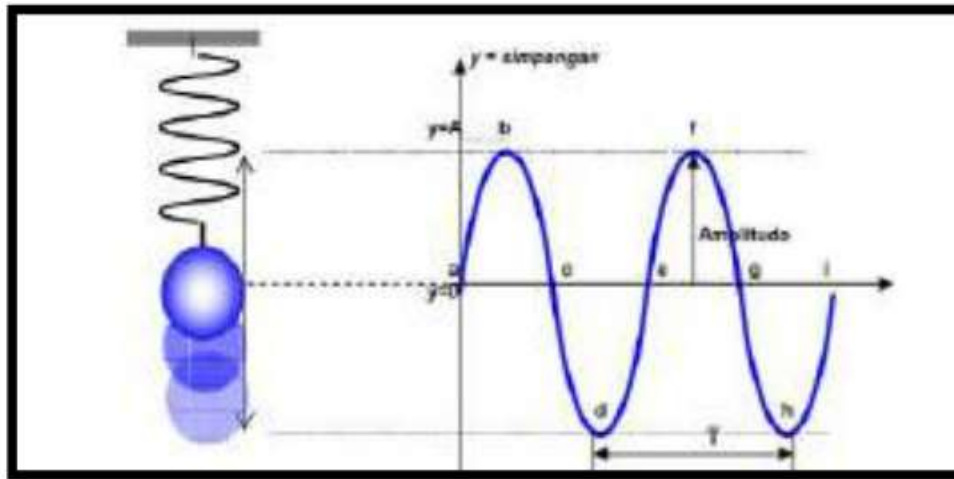
Gambar 4.4. Anatomi Gerak Harmonik Sederhana pada Pegas
