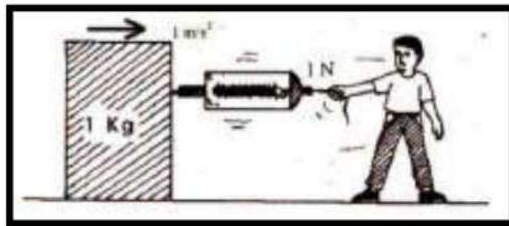
Gambar 4.8. Gaya Satu Newton
