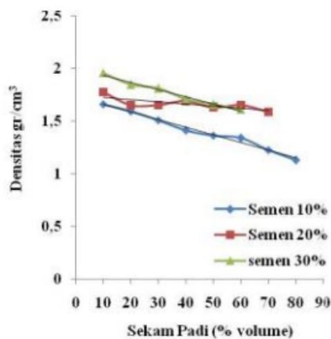
Gambar 5. 11 Grafik hasil uji densitas
