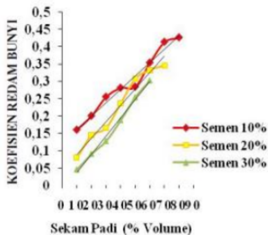
Gambar 5. 14 Grafik hasil uji serap suara
