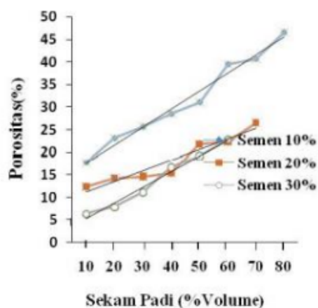
Gambar 5.12 Grafik hasil uji porositas
