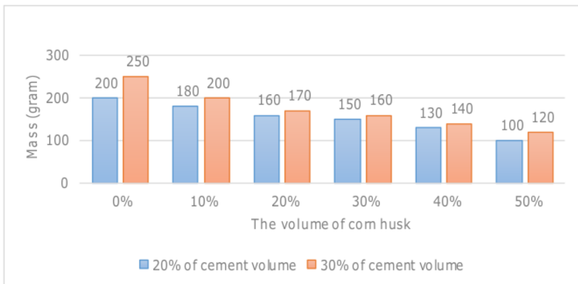
Gambar 5.3 Grafik massa batako ringan
