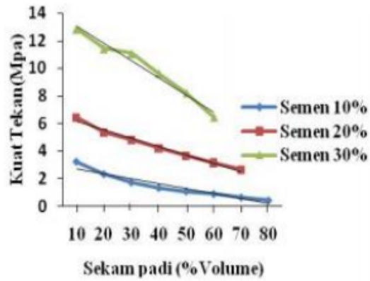
Gambar 5.13 Grafik hasil uji tekan
