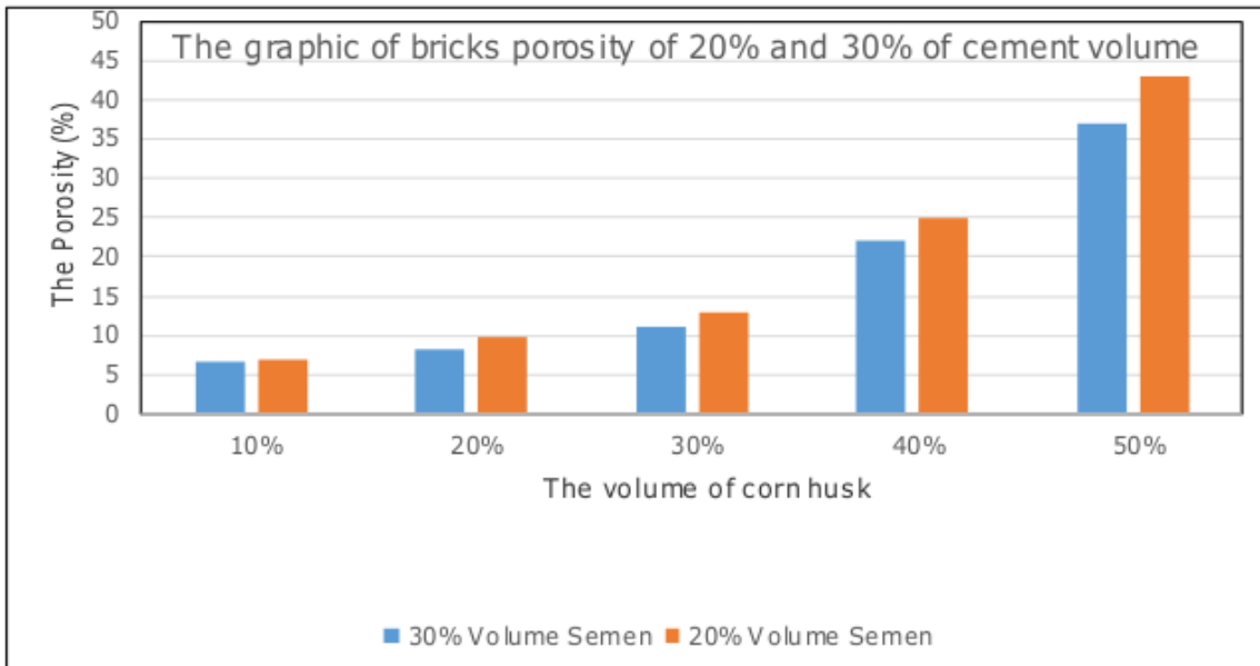
Gambar 5.6 Grafik porositas batako ringan 20% dan 30% volume semen
