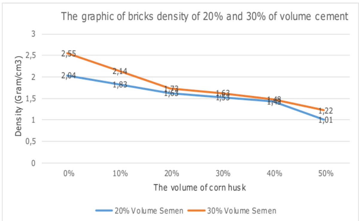
Gambar 5.4 Grafik densitas batako 20% dan 30% Volume semen
