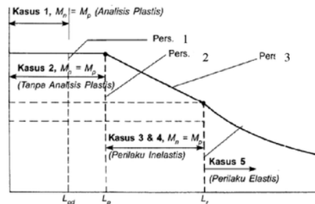
Gambar 1. Kuat momen nominal akibat tekuk torsi lateral
