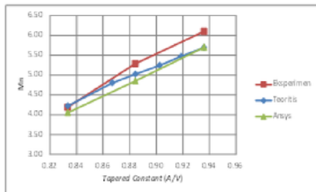
Gambar 14. Kurva hubungan tapered constant dan momen kapasitas M_n untuk berbagai model pada pengujian teoritis, eksperimen, dan ANSYS.
