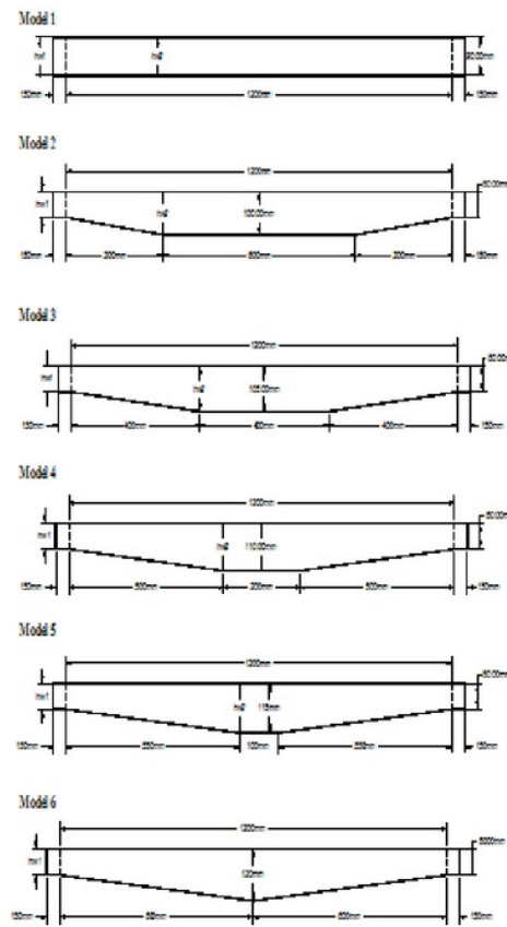
Gambar 7. Model dan ukuran benda uji
