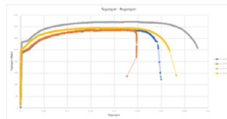
Gambar 9. Kurva hubungan Tegangan-regangan
