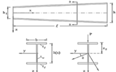
Gambar 2. Karakteristik geometrik dari tapered I-beam
