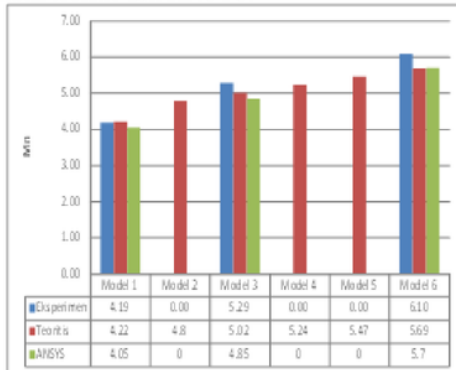
Gambar 13. Diagram batang kapasitas lentur dari berbagai model pada pengujian teoritis, eksperimen, dan ANSYS
