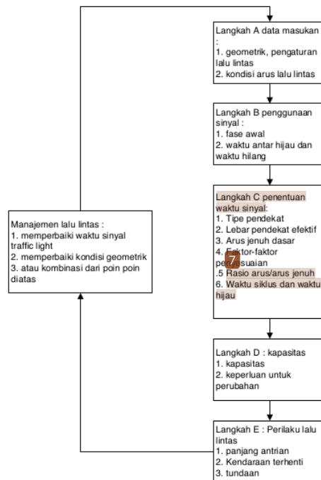
Gambar 4 Diagram Alir Perhitungan Simpang Bersinyal
