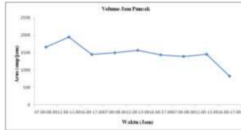
Gambar 6 Grafik Volume Jam Puncak Simpang Tugu Pecel Arus tertinggi untuk simpang Tugu Pecel yaitu 1945 smp/jam.
