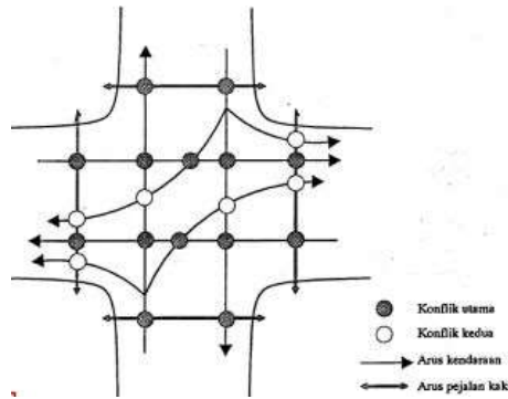
Gambar 1 Konflik Lalu Lintas Pada Simpang Empat Lengan
