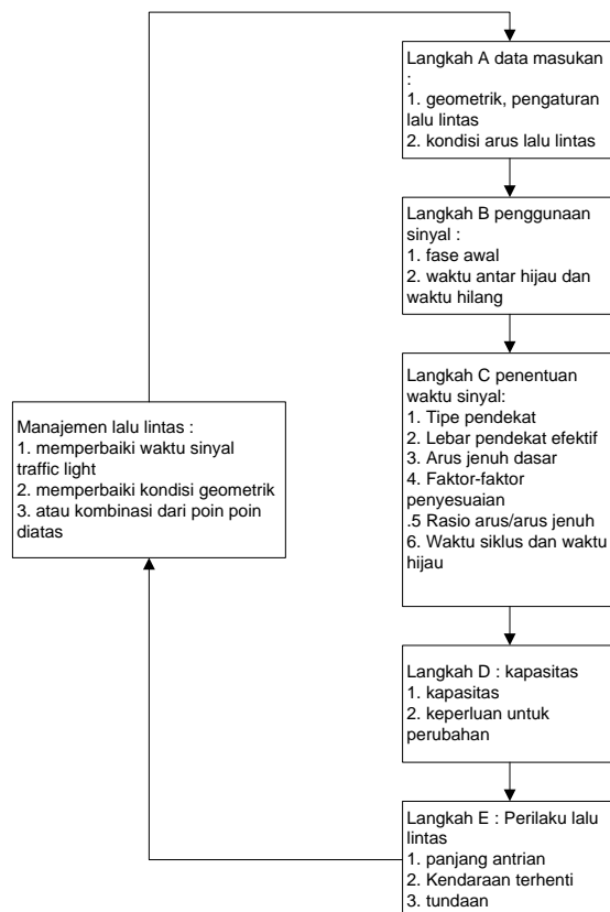
Gambar 4 Diagram Alir Perhitungan Simpang Bersinyal
